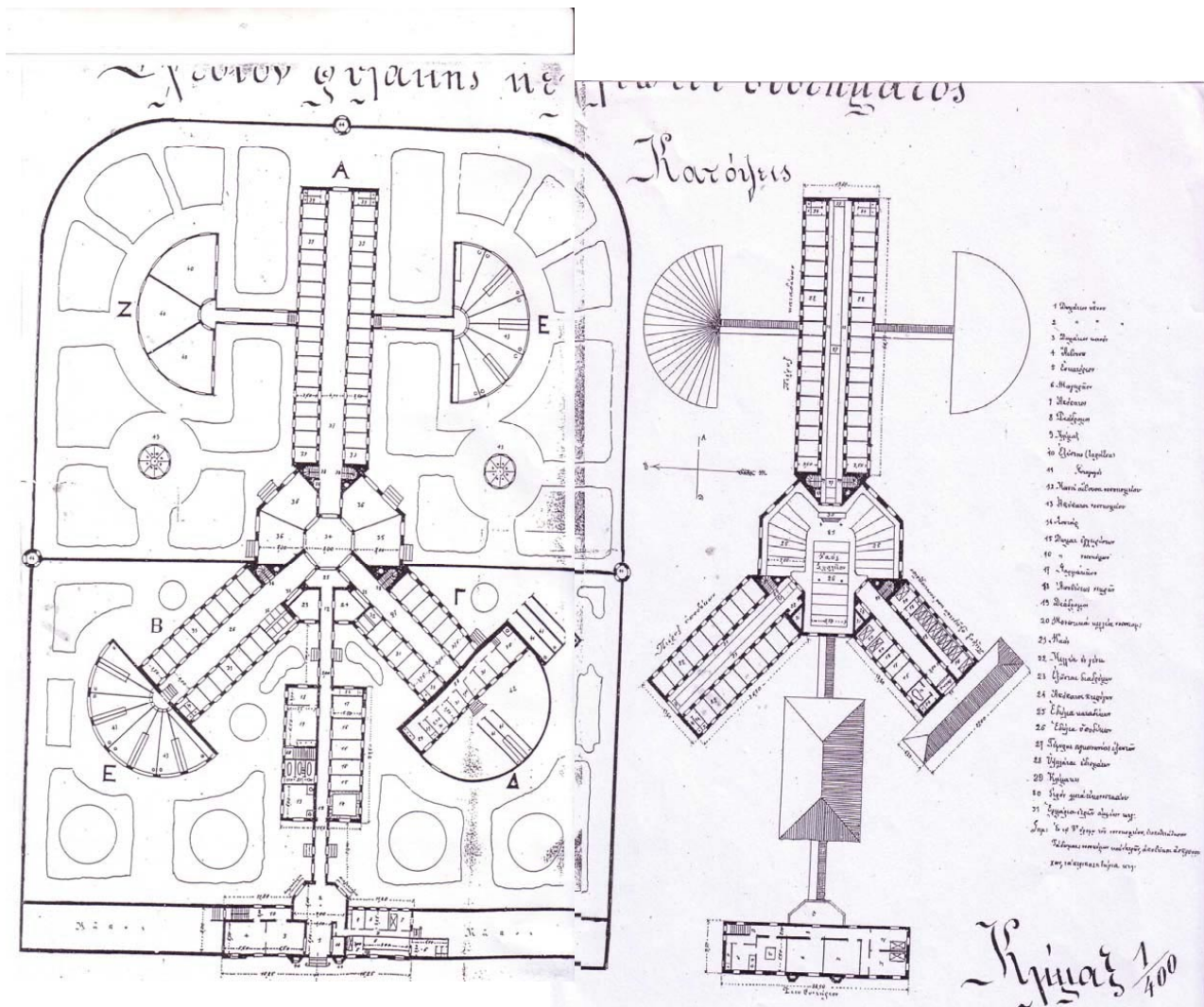
Σχήμα 7: Σχέδιο φυλακής απομονωτικού συστήματος από το Αντωνίου Μαναράκη (νομομηχανικού), Μελέτη περί οικοδομής φυλακών απομονωτικού και μικτού συστήματος μετά διαγραφμάτων. Επί τη βάσει του νομοσχεδίου της επιτροπής του Υπουργείου της Δικαιοσύνης, Αθήνα, 1900.
