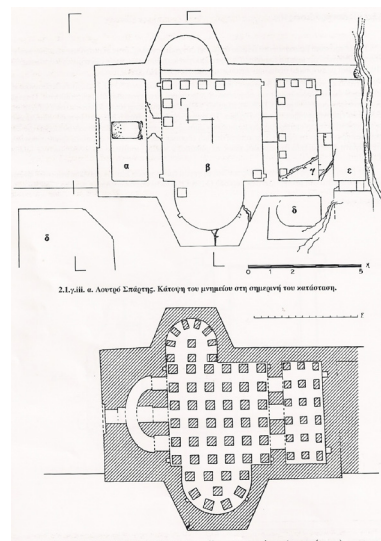
Εικ.41: Λουτρό Σπάρτης. Κάτοψη ισογείου και στη στάθμη των υποκαύστων (πηγή: Ελένη Κανετάκη, Οθωμανικά Λουτρά στον Ελλαδικό Χώρο, σελ. 34)
