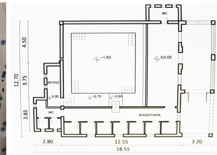
Εικ.74: πάνω: Κάτοψη ισογείου, Λουτρά Λαγκαδά Εικ.75: κάτω αριστερά: Τοπογραφικό λουτρικού συγκροτήματος Λαγκαδά Εικ.76: κάτω δεξιά: Κάτοψη ισογείου του αμμόλουτρου Λαγκαδά (πηγή: Διπλωματική Εργασία Χριστίνας Παπακώστα, Αναβάθμιση και εκσυγχρονισμός των ιαματικών εγκαταστάσεων στο Λαγκαδά Θεσσαλονίκης, Φεβρουάριος 2010)
