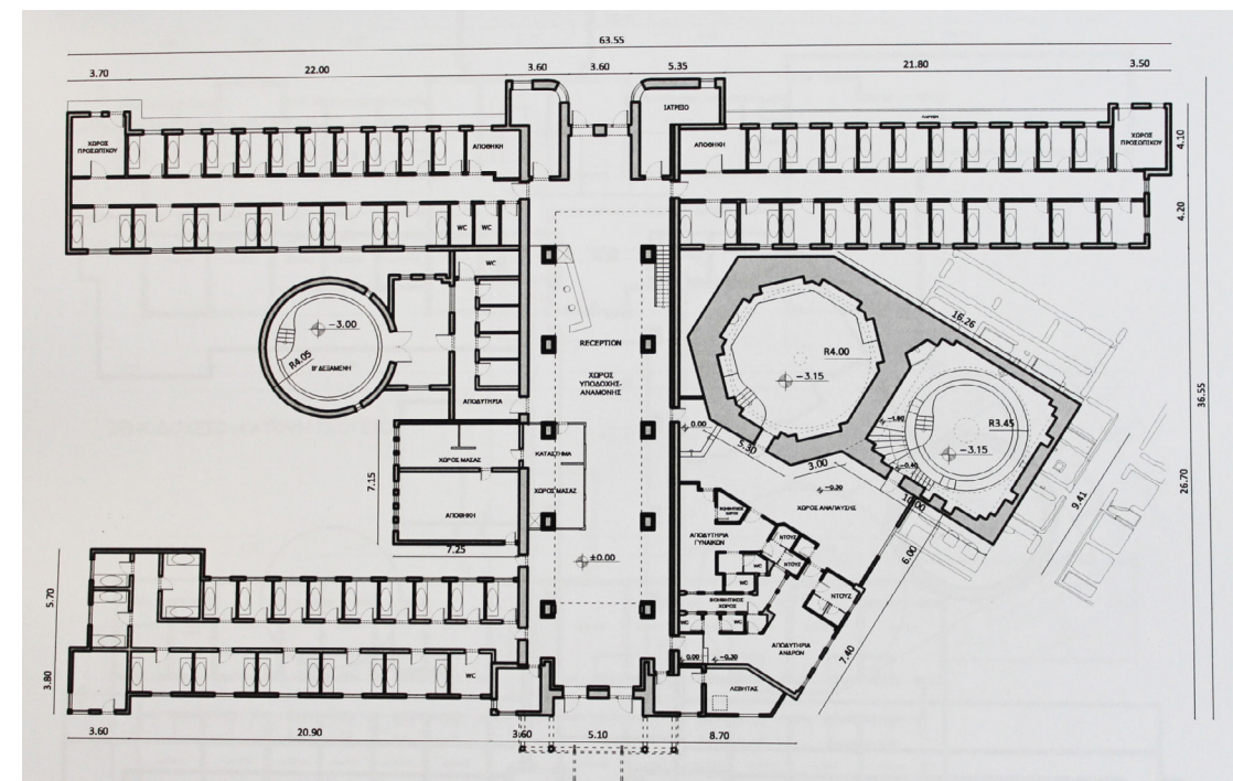
Εικ.74: πάνω: Κάτοψη ισογείου, Λουτρά Λαγκαδά Εικ.75: κάτω αριστερά: Τοπογραφικό λουτρικού συγκροτήματος Λαγκαδά Εικ.76: κάτω δεξιά: Κάτοψη ισογείου του αμμόλουτρου Λαγκαδά (πηγή: Διπλωματική Εργασία Χριστίνας Παπακώστα, Αναβάθμιση και εκσυγχρονισμός των ιαματικών εγκαταστάσεων στο Λαγκαδά Θεσσαλονίκης, Φεβρουάριος 2010)
