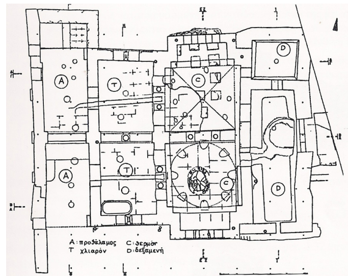
Εικ.40: Κάτοψη του Λουτρού Κουλέ Καφέ στην Θεσσαλονίκη (πηγή: Ελένη Κανετάκη, Οθωμανικά Λουτρά στον Ελλαδικό Χώρο, σελ. 29)
