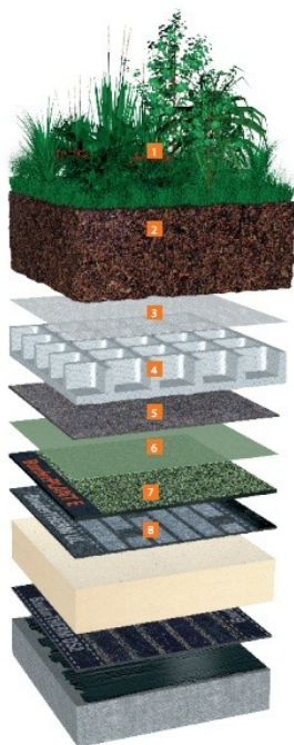
Εικόνα 3.2, Στρώσεις εκτατικού τύπου φυτεμένου δώματος, (Πηγή: http://www.karteco.gr )
