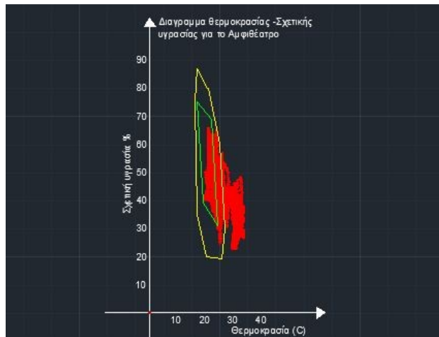
Εικόνα 9.6, Διαγραμμα θερμοκρασίας υγρασίας για το Αμφιθέατρο από τις μετρήσεις των θερμουγρομέτρων
