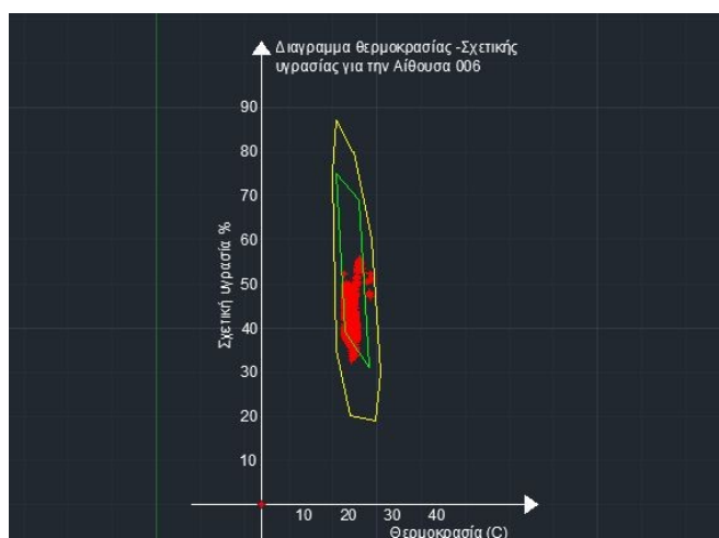
Εικόνα 9.2, Διαγραμμα θερμοκρασίας υγρασίας για την Αίθουσα 006 από τις μετρήσεις των θερμογρομέτρων
