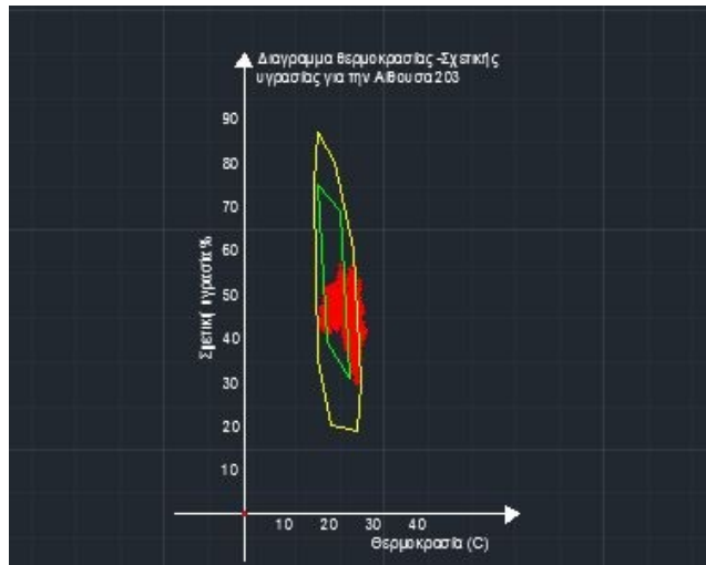
Εικόνα 9.17, Διαγράμμα θερμοκρασίας υγρασίας για την Αίθουσα 203 τις μετρήσεις των θερμογρομέτρων
