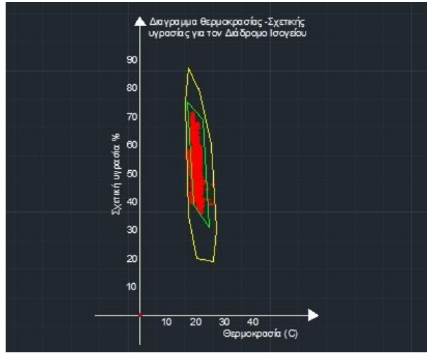
Εικόνα 9.4, Διαγραμμα θερμοκρασίας υγρασίας για τον Διαδρομο Ισογείου από τις μετρήσεις των θερμουγρομέτρων
