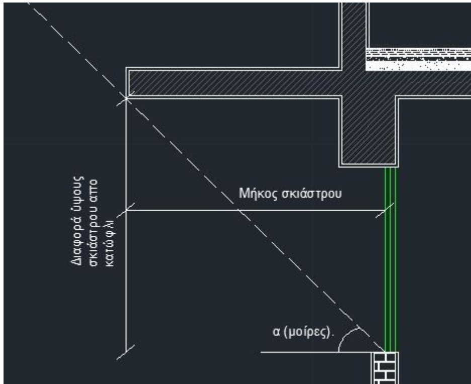
Εικόνα 10.32, Υπολογισμός κατάλληλου μήκους οριζόντιου σκιάστρου
