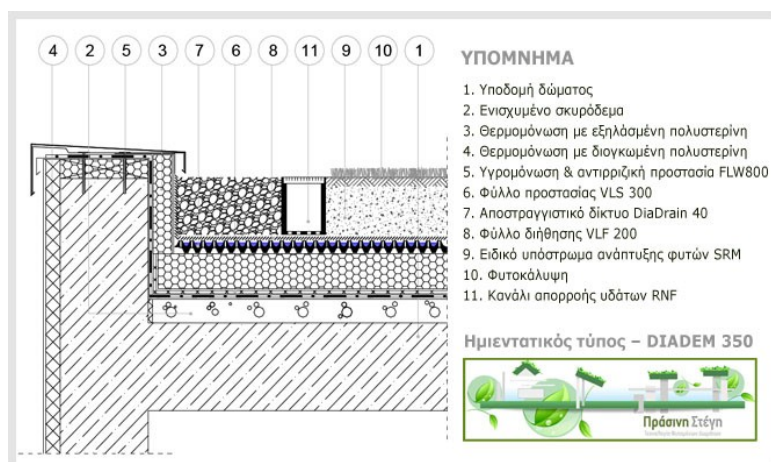
Εικόνα 3.4, Στρώσεις ημιεντατικού τύπου φτεμένου δώματος, (Πηγή: http://www.prasinistegi.gr )
