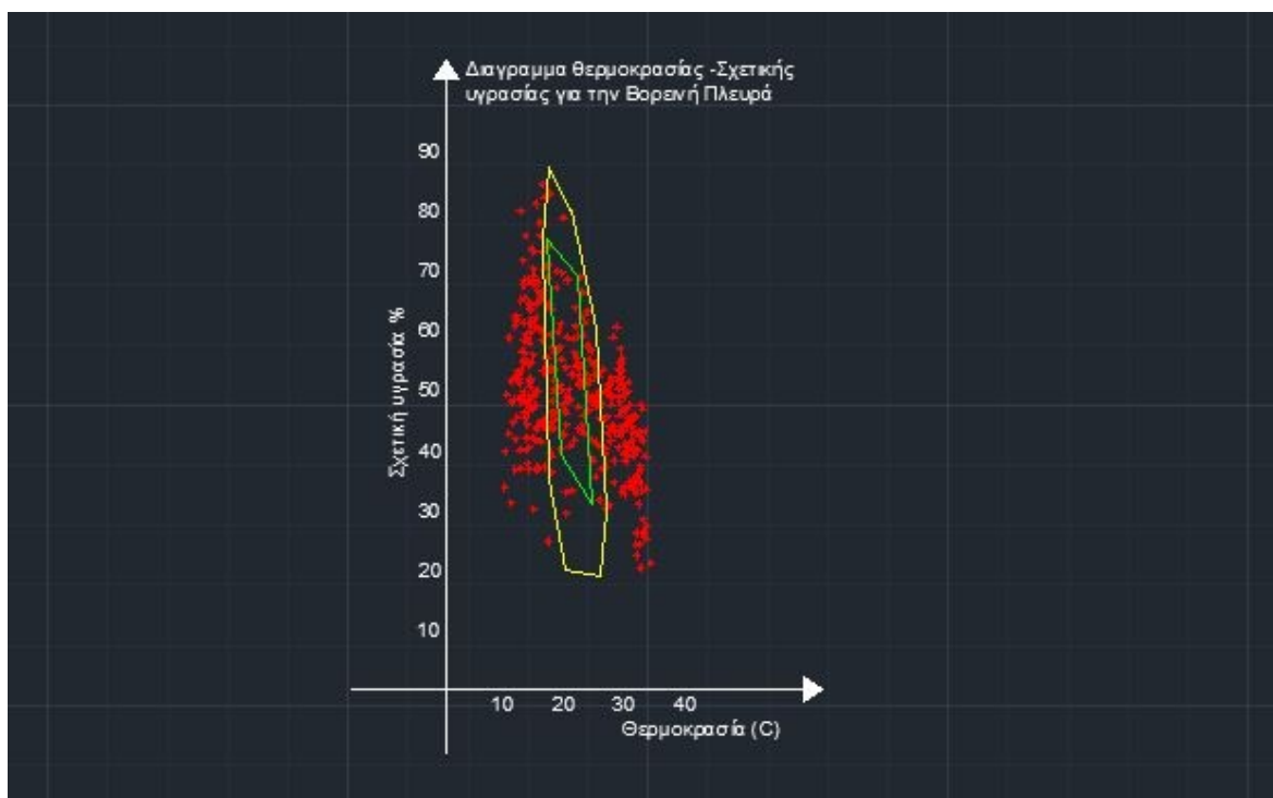
Εικόνα 6.18, Διάγραμμα θερμοκρασίας – Σχετικής υγρασίας για τη Βόρεια πλευρά
