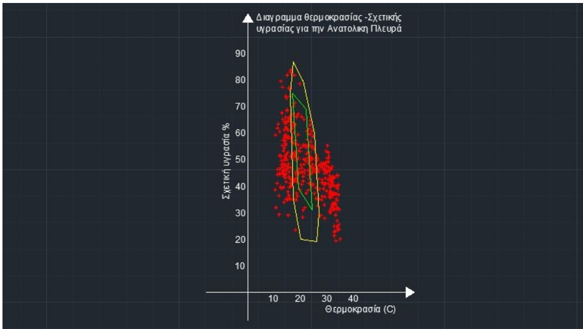
Εικόνα 6.17, Διάγραμμα θερμοκρασίας – Σχετικής υγρασίας για την Ανατολική πλευρά
